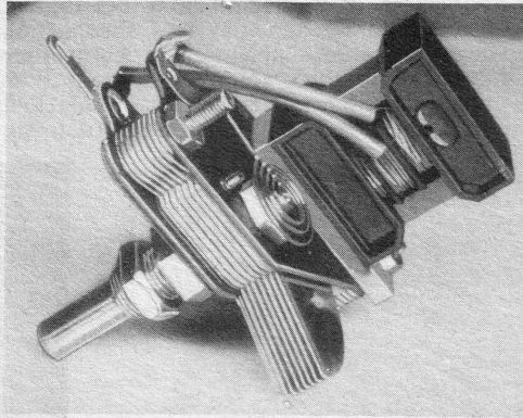
Der kleine Sperrkreis in Schaltung und Ansicht. Die Spule ist unmittelbar am Drehko befestigt. (Aufn. vom Verfaßer)
