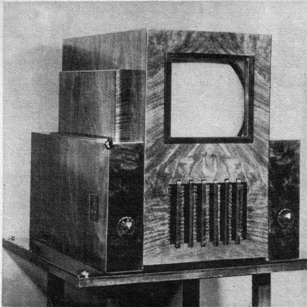
Die Frontansicht des Loewe-Fernsehers FEB. Unter dem vier-eckigen Gehäuseausschnitt, hinter dem sich die weiße Fläche befindet, auf der das Fernsehbild zu sehen ist, sitzt der Lautsprecher. Links und rechts die Bedienungsköpfe. Das Ganze ist nur etwa doppelt so schwer als ein Groß-Superhet. (Werkphoto)
