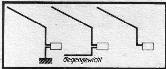
Abb. 1. Drei Hochantennen-Anlagen. Die erste erhält ihre Spannung zwischen Antenne und Erde. In der zweiten Anlage ist die Erdung durch ein Gegengewicht ersetzt. In der dritten Anlage bildet das Gerätegestell selbst das Gegengewicht.
