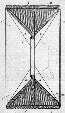
Abb. 2. Ein Längsschnitt durch den „Kastentonnfreien“.
