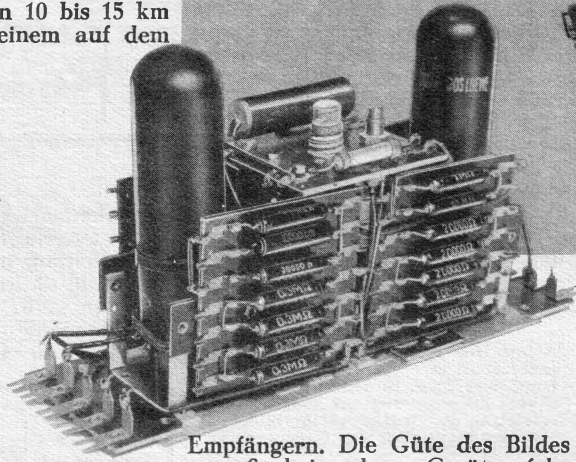
Drei Bausteine des Fernsehers. Sie sind so gebaut, daß sie gegenseitig auswechselbar einen Block für sich bilden. (Werkphoto Radiogef. D. S. Loewe)
