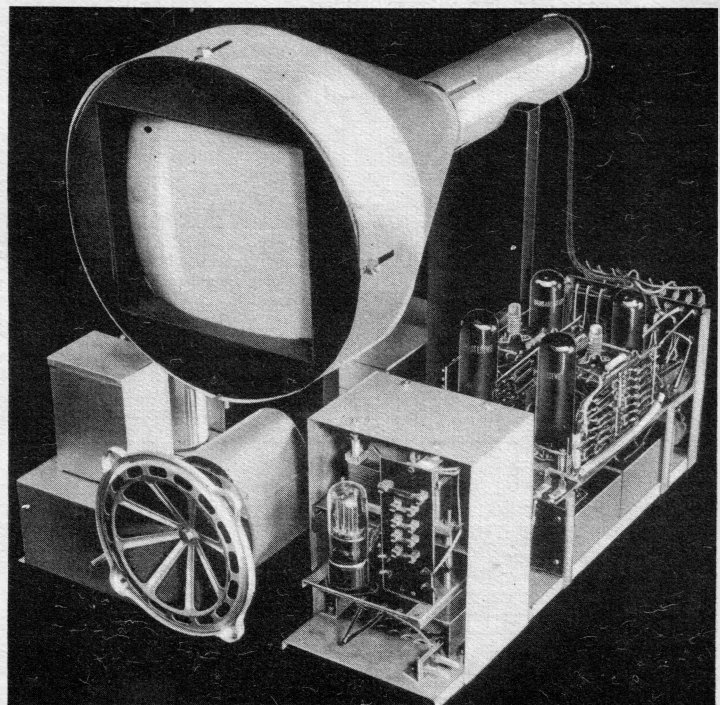
Die Innenansicht des Loewe-Fernsehers FEB. Die Fernfehröhre ist zum Schutze gegen Beschädigungen von einem Metallmantel umgeben. (Werkphoto)
