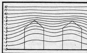
Abb. 8. Die Spannungslinien für zwei nebeneinander stehende Häuser, die kein Blechdach aufweisen. Die Häuser sind als etwas leitend angenommen, wobei die Leitfähigkeit nach dem Inneren hin zunimmt. Auf die einzelnen Metallteile und Leitungen des Hauses ist keine Rücksicht genommen, da deren Anordnungen in jedem Einzelfall wieder andere sind. Wir erkennen, daß auch in dem Zwischenraum zwischen den beiden Häusern eine erhebliche Feldverzerrung zustande kommt.
