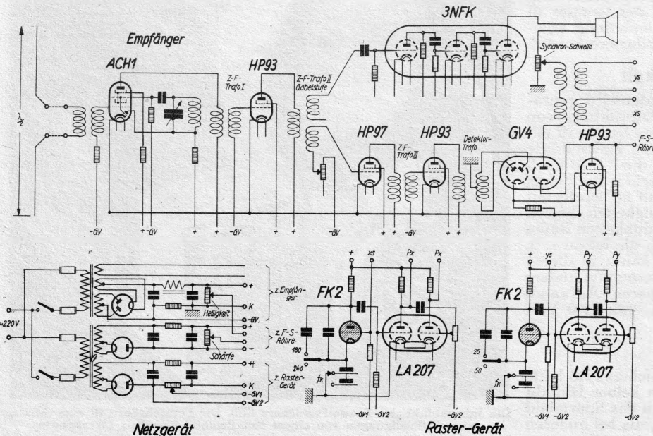
Ein vereinfachtes Schaltbild. Die Mifchung und ZF-Verstärkung erfolgt für Bild- und Tonwelle gemeinsam, hinter der letzten ZF-Stufe findet die Gabelung statt, und Ton und Bild gehen nun ihre eigenen Wege.
