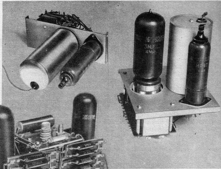
Drei Bausteine des Fernsehers. Sie sind so gebaut, daß sie gegenseitig auswechselbar einen Block für sich bilden. (Werkphoto Radiogef. D. S. Loewe)
