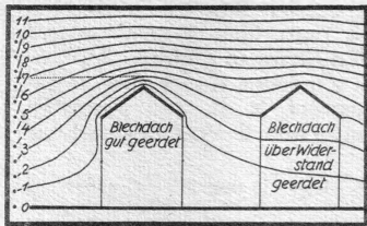
Abb. 9. Blechdächer können das am Empfangsort vorhandene Senderfeld außerordentlich stark verzerrern. Die Verzerrung ist bei guter Erdung des Blechdaches besonders stark. Die punktierte Linie auf der linken Seite bringt zum Ausdruck, daß über dem Dachfirst — infolge der vom geerdeten Blechdach herrührenden Verzerrung — an Stelle der Spannungszahl 7,5 nur die Spannungszahl 3,5 auftritt.
